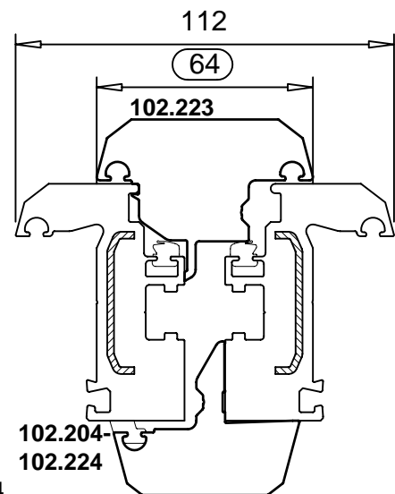
Flügelverstärkung weiß & farbig - 113.291 - Ix = 1,90cm 4
